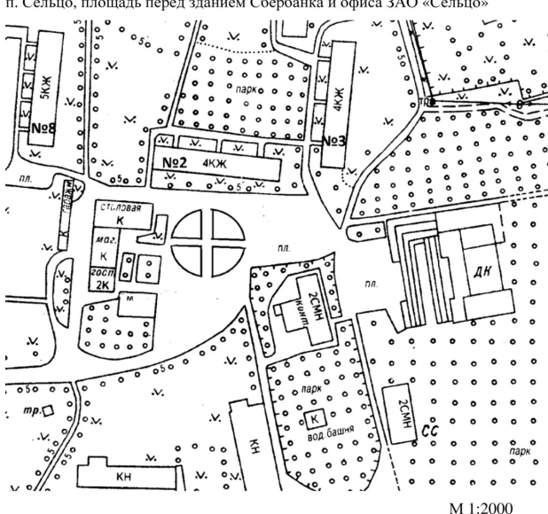
Графическое изображение НТО с идентификационным № 2
